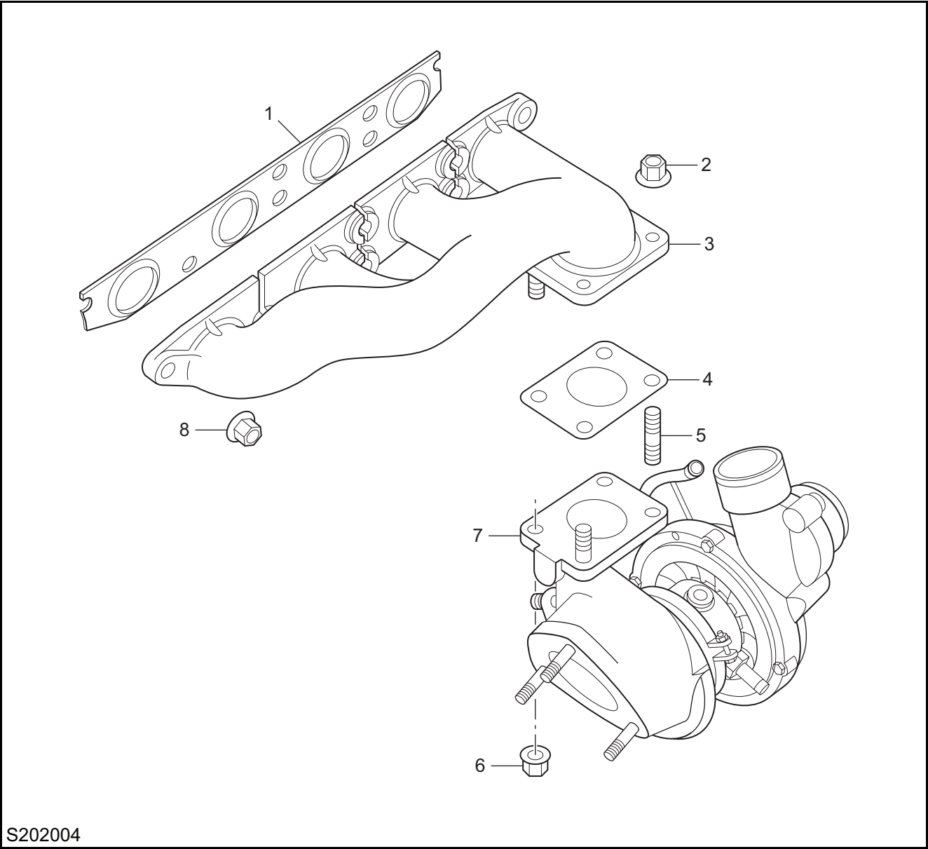
排气歧管分解图 — 涡轮增压发动机
