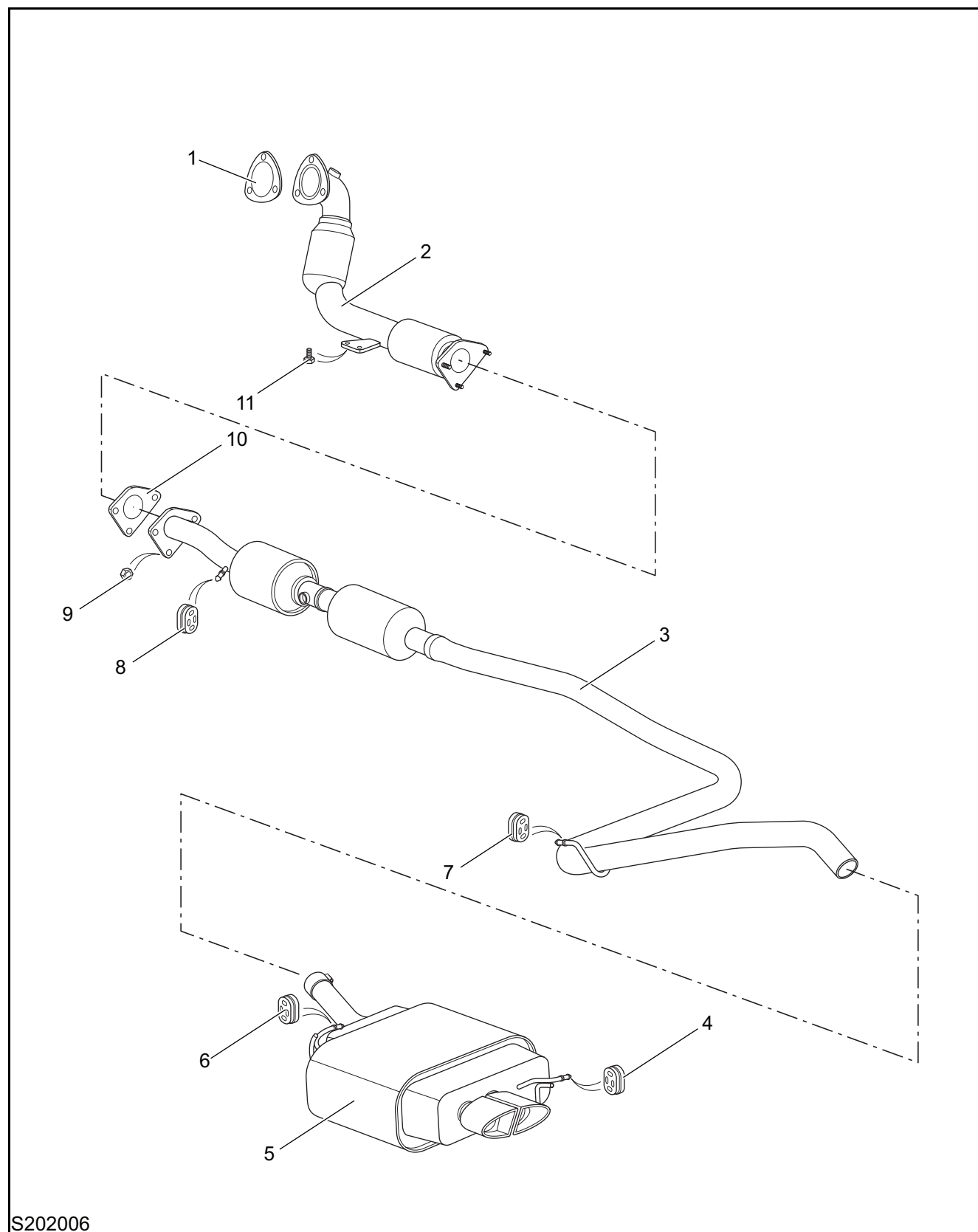
排气系统分解图— 涡轮增压发动机
