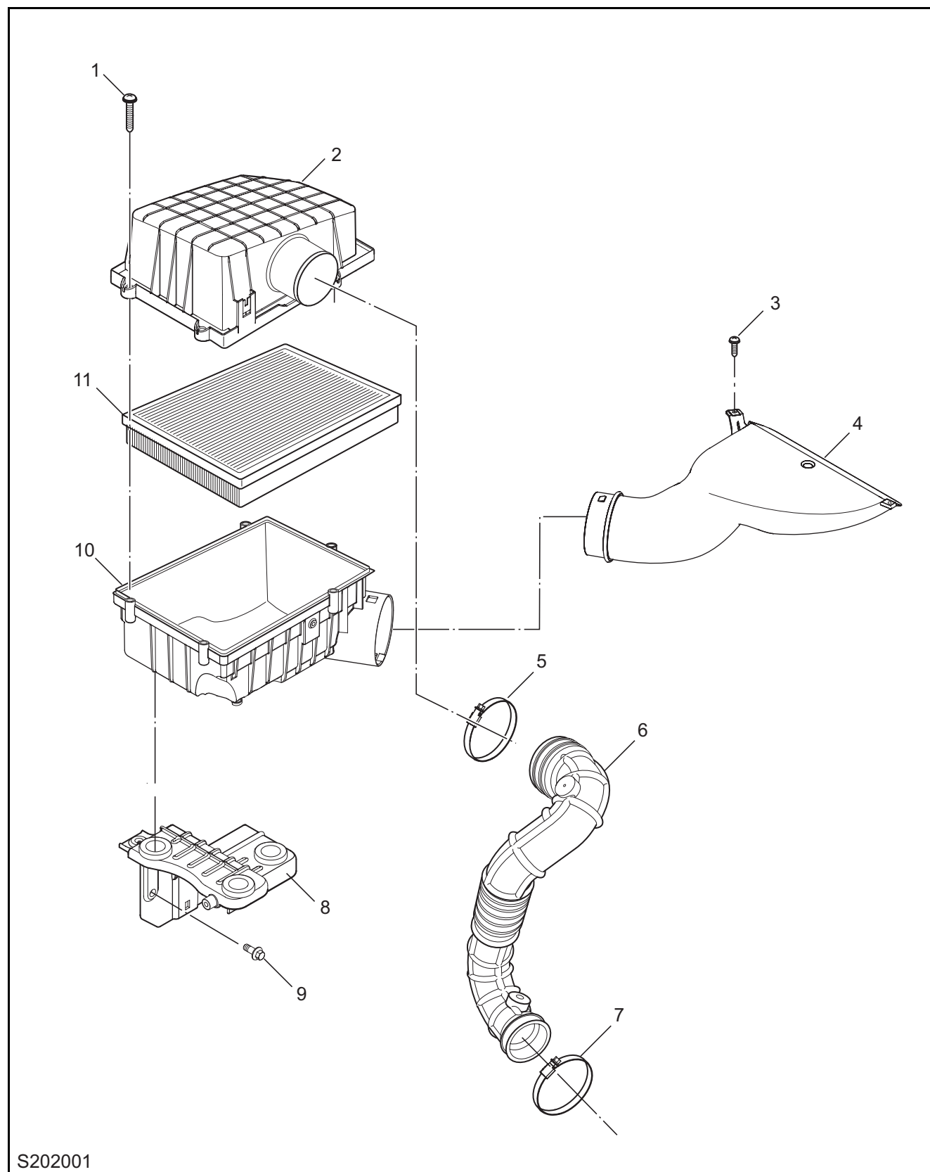
空气滤清器分解图 — 涡轮增压发动机
